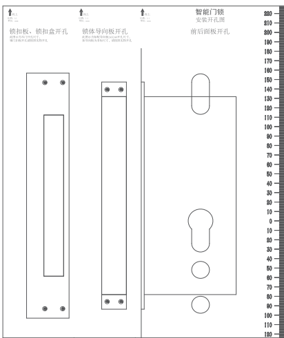
开孔模板
