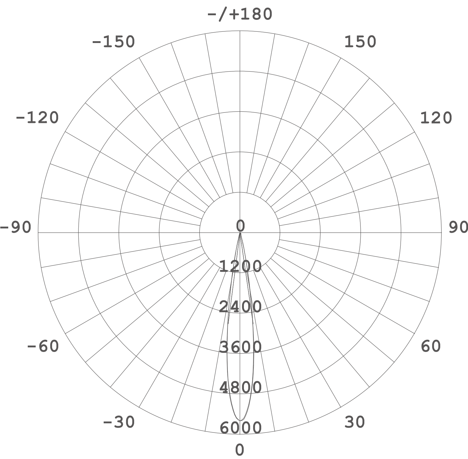
平均光束角: 15°
