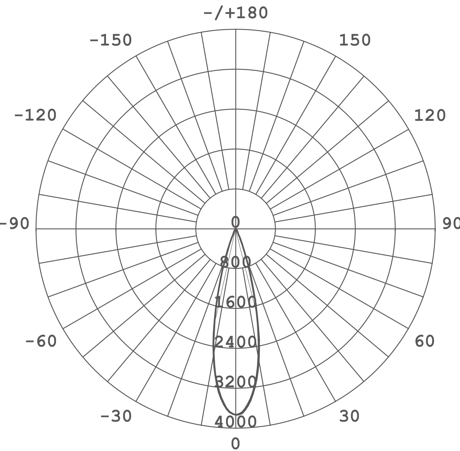
平均光束角: 24°
