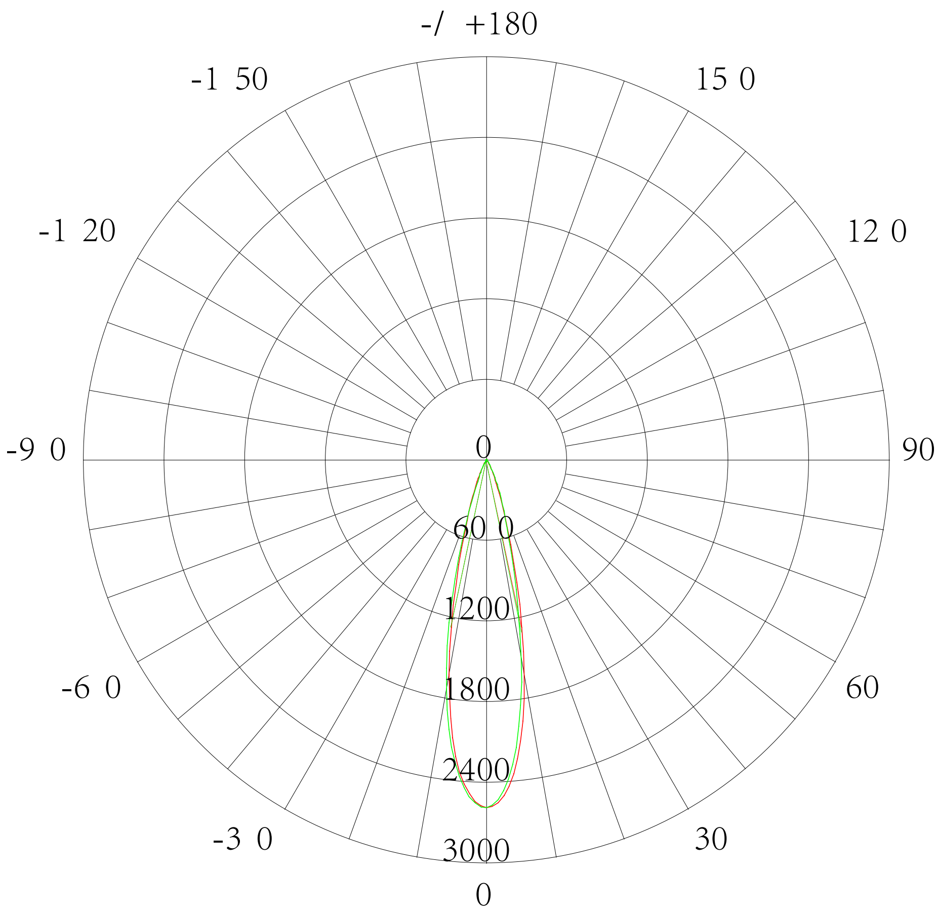
平均光束角：24°
