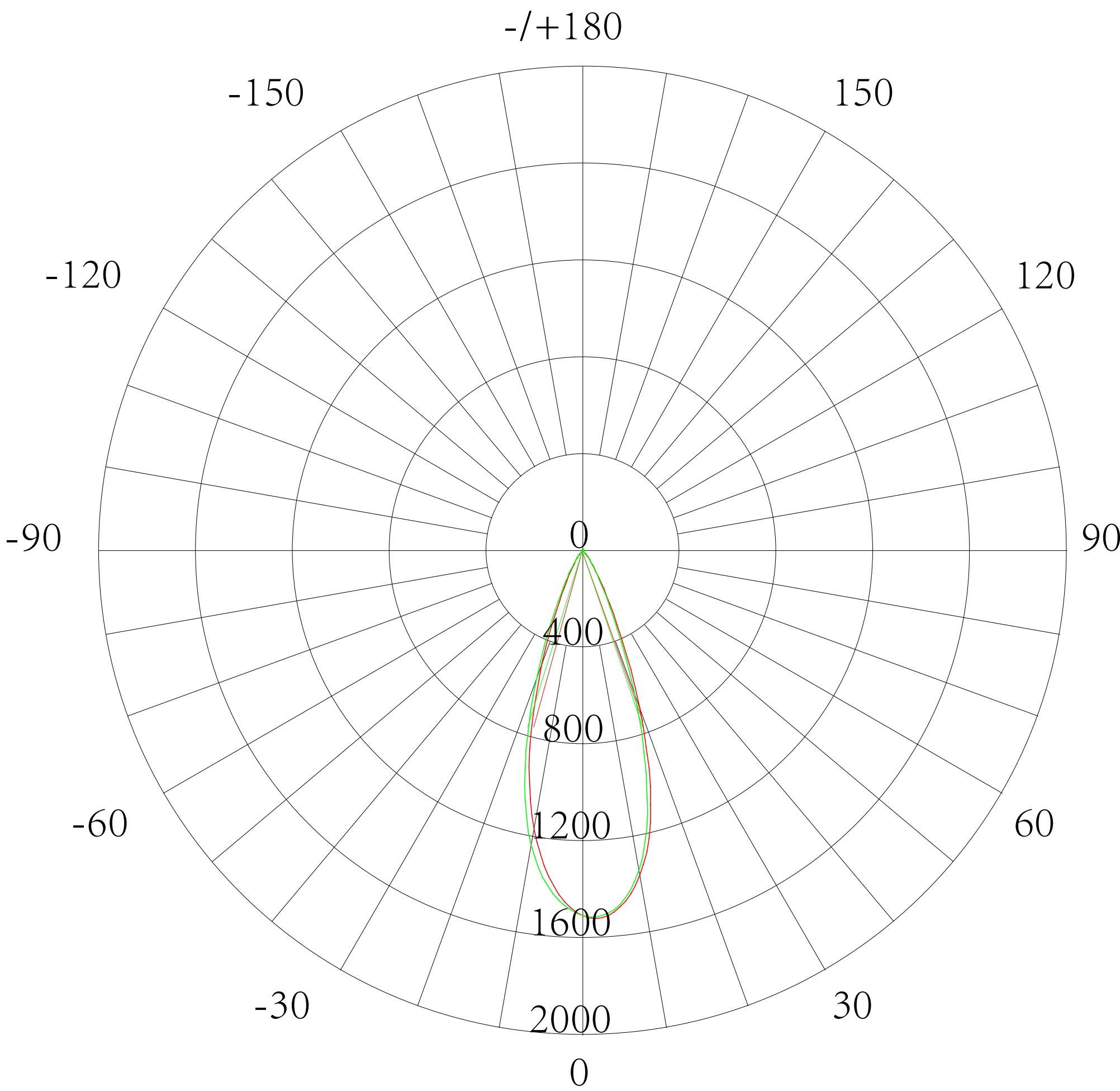
平均光束角：36°
