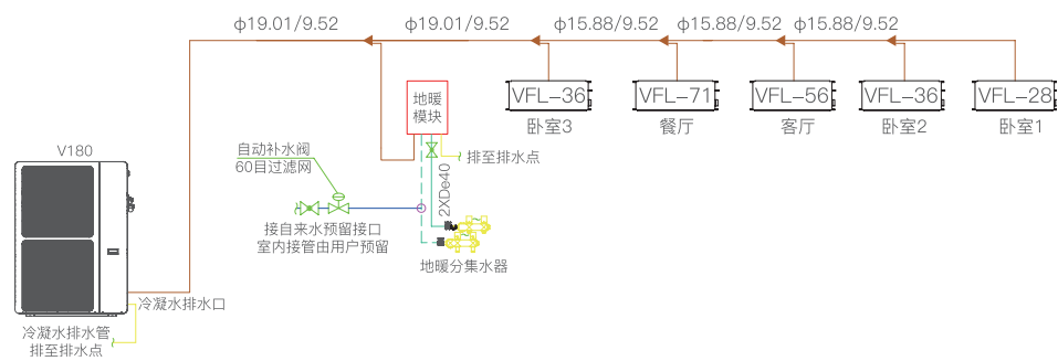
V180 主机（搭配地暖模块）工程应用示意图：
