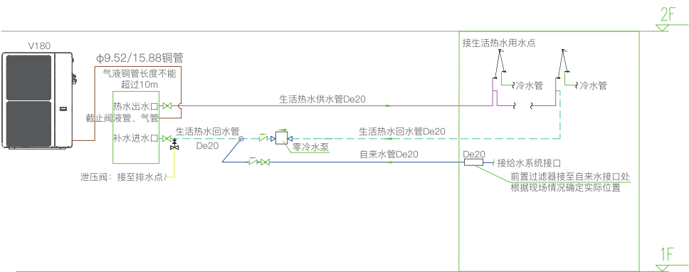
V180 主机（搭配热水模块）工程应用示意图：
